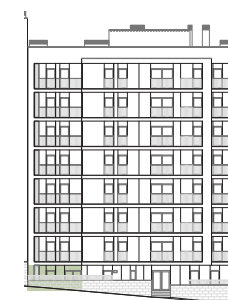
ALÇADO NASCENTE EAST FACADE FAÇADE EST
